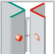
3 renforts de paumelles soudés
