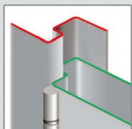
Anti-dégondage par tenon-mortaise
