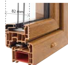
RENFORCEMENT SUR OUVRANT AVEC FIBRES TRESSÉES EN CONTINU ET DORMANT AVEC UN RENFORT ACIER (SUIVANT ABAQUE POUR LE BLANC, BEIGE ET GRIS ET SYSTÉMATIQUE POUR L'ASPECT BOIS). APPORTE RIGIDITÉ ET TENUE DANS LE TEMPS SANS AUCUN DÉRÈGLEMENT DES OUVRANTS
